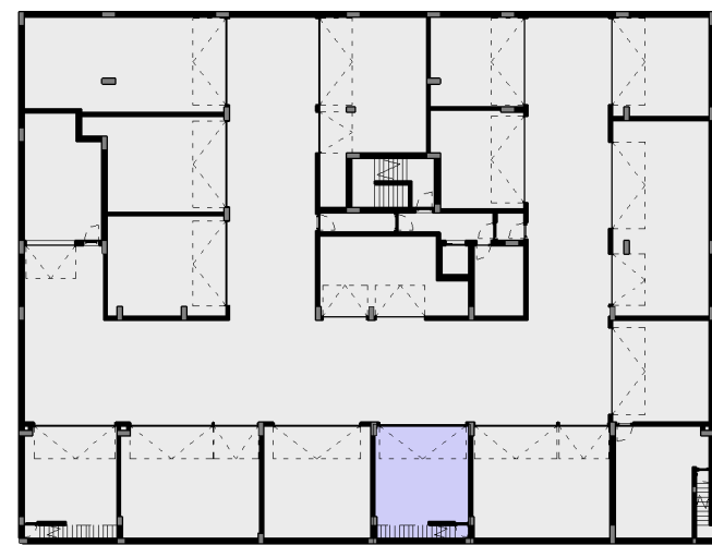
E - BOX / ESTACIONAMENTO 1:500
