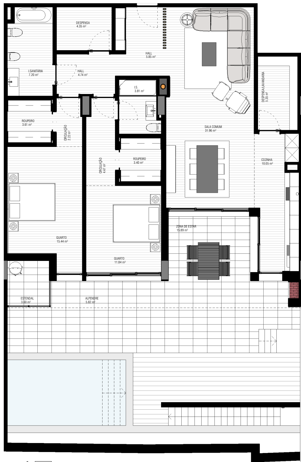
E - FRACÇÃO 1:100
