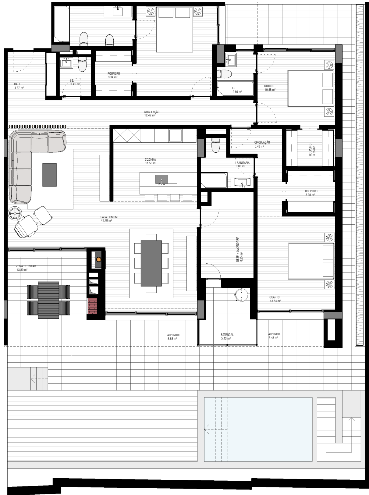
F - FRACÇÃO 1:100
