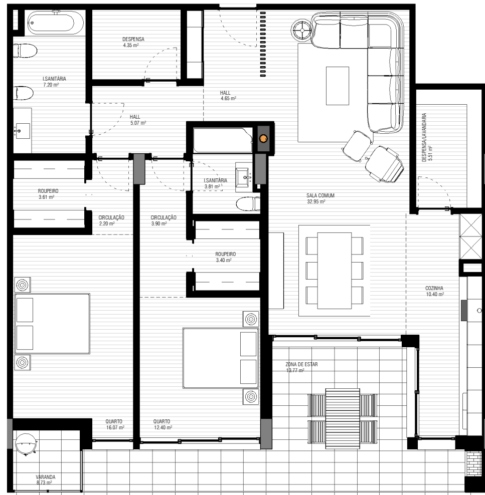
K - FRACÇÃO 1:100
