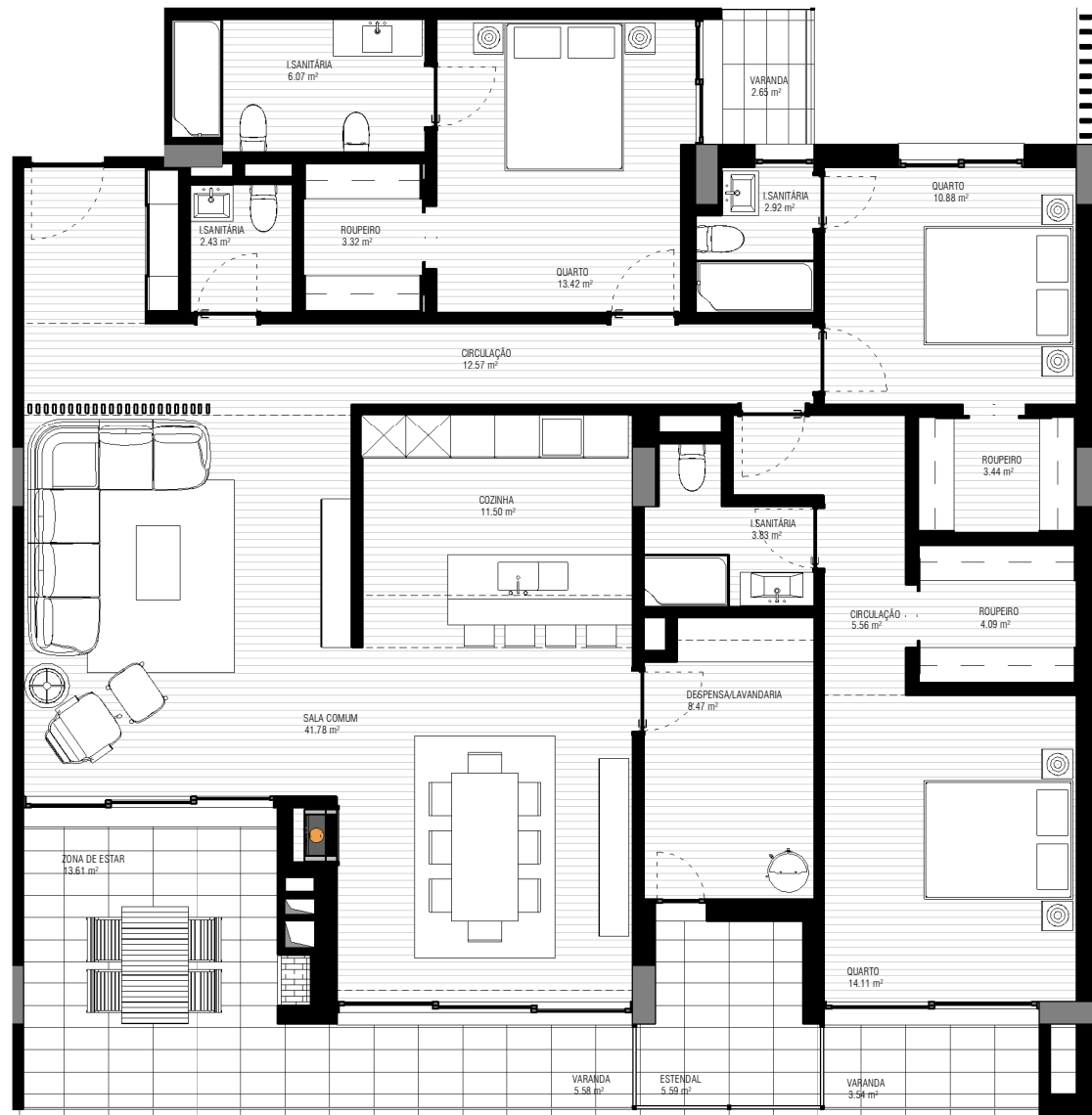
L - FRACÇÃO 1:100
